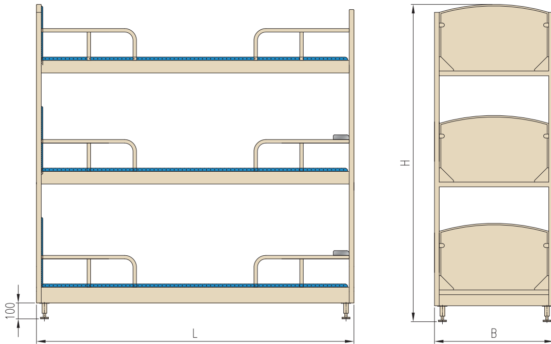
图3/ 单层软垫柜床 (左式) 结构示意图
