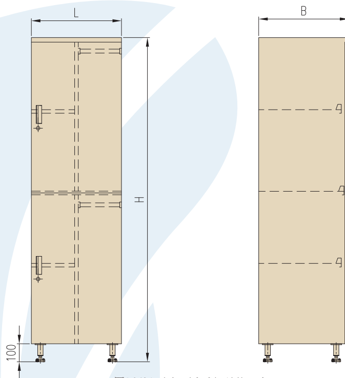
图2/ 单门衣柜（右式）结构示意图
