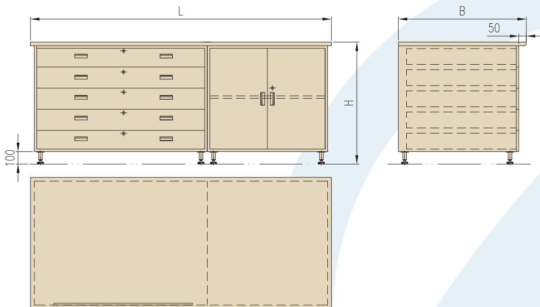
图4/ 海图桌（J240型）结构示意图
