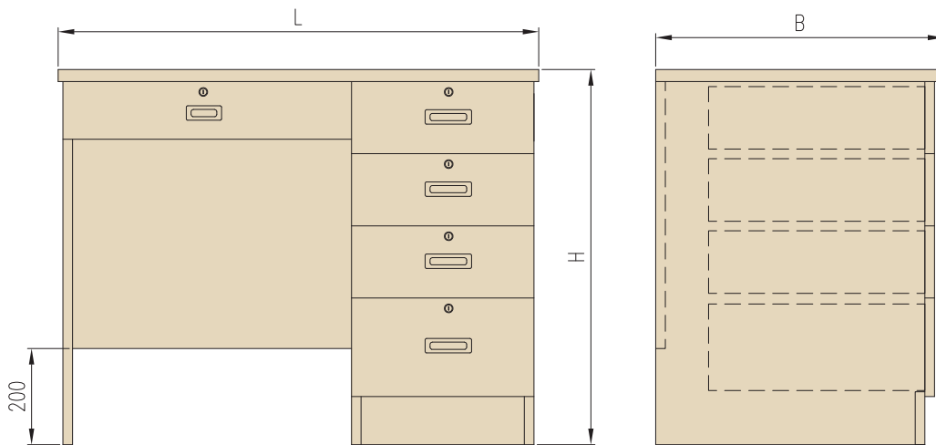
图1/ 单台座办公桌（左式）结构示意图
