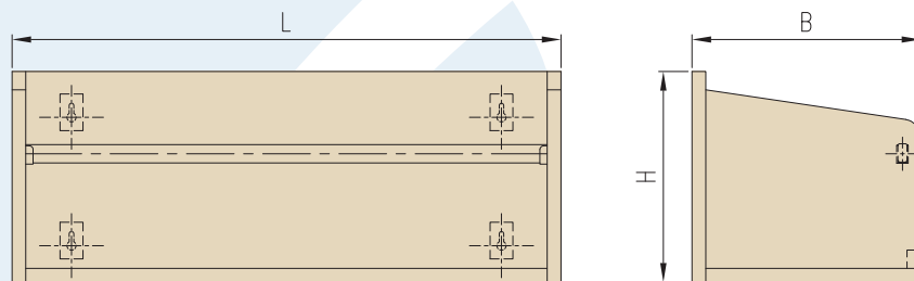
图6/ 书架（P型）结构示意图
