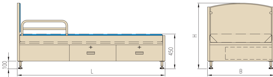
图1/ 单层软垫柜床（左式）结构示意图
