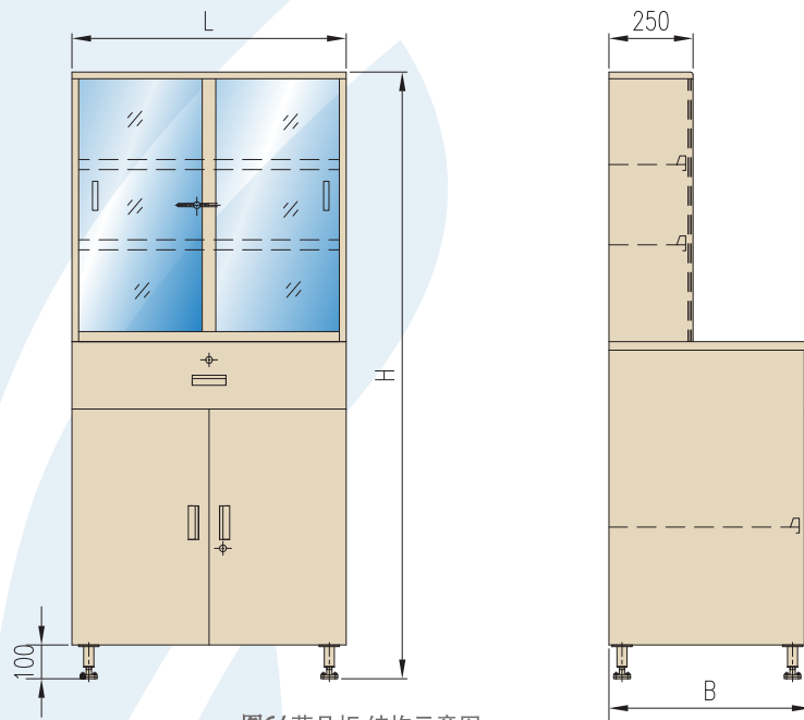
图6/ 药品柜 结构示意图
