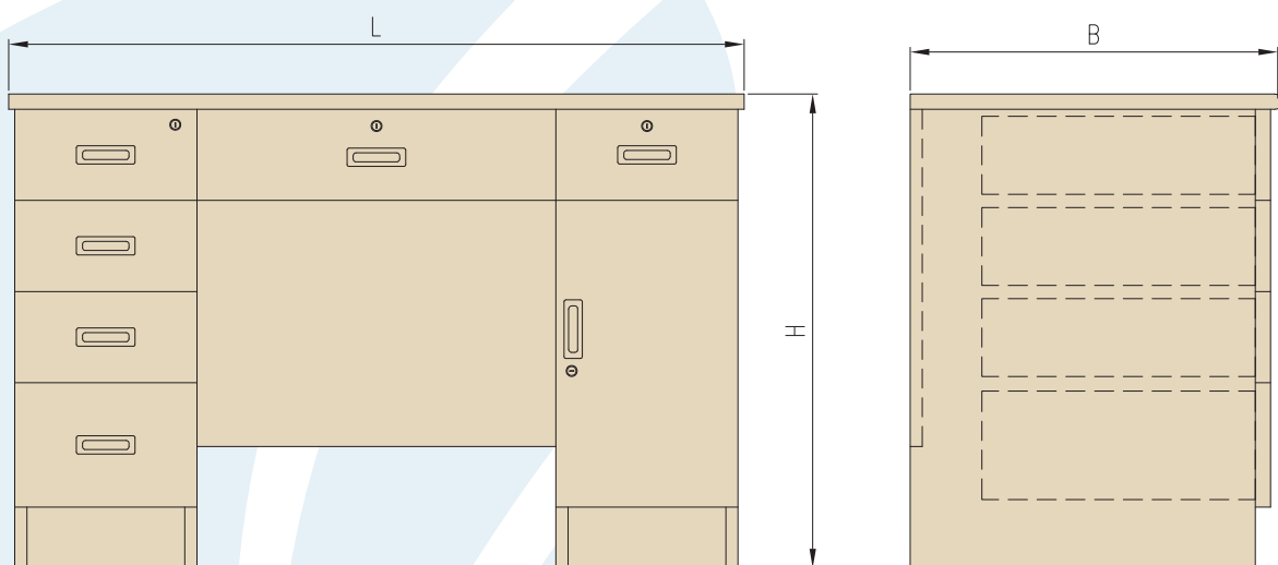
图2/ 双台座办公桌 结构示意图
