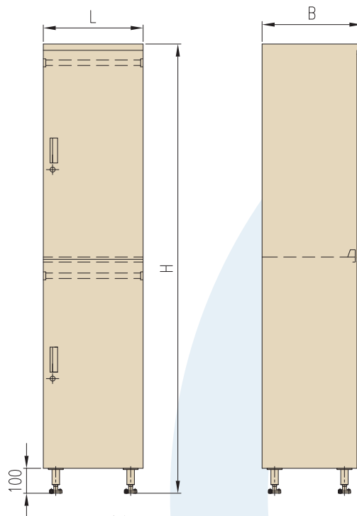
图4/ 更衣柜 结构示意图
