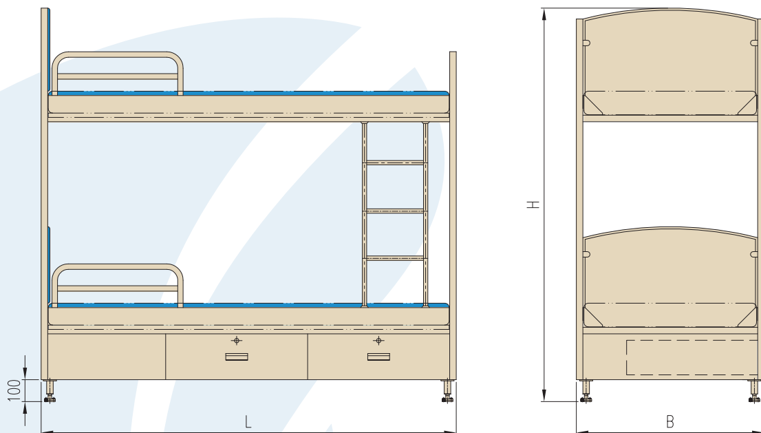
图2/ 双层柜床（左式）结构示意图
