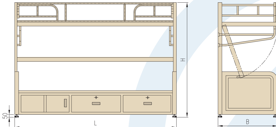
图4/ 沙发床 (左式) 结构示意图
