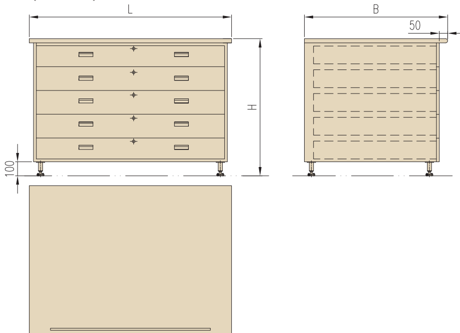
图3/ 海图桌（J141型）结构示意图
